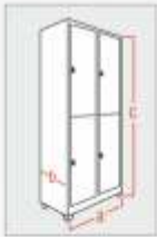
4'lü Dolap Ölçüleri 4-Lockers dimensions
